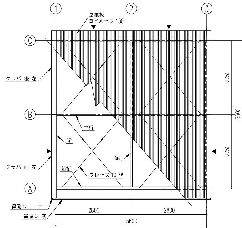
小屋伏図 (S=1/80)
