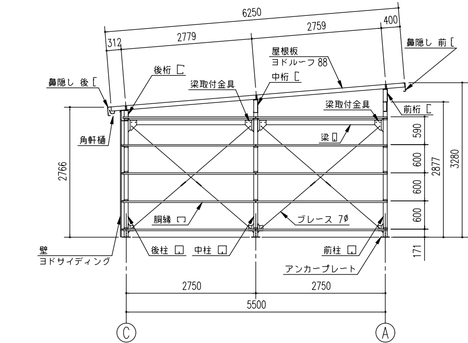
側面断面図 (S= 1/80)
