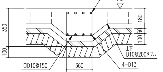
C ~ C' 断面
