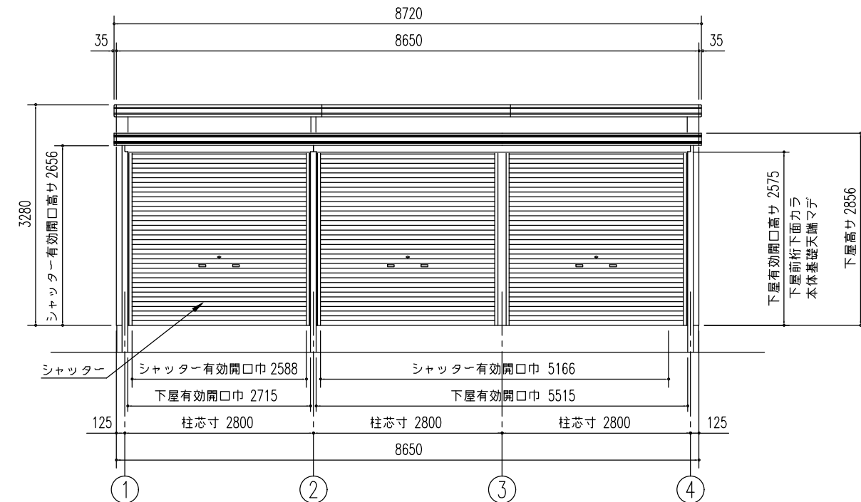
正面立面図(S=1/80)
