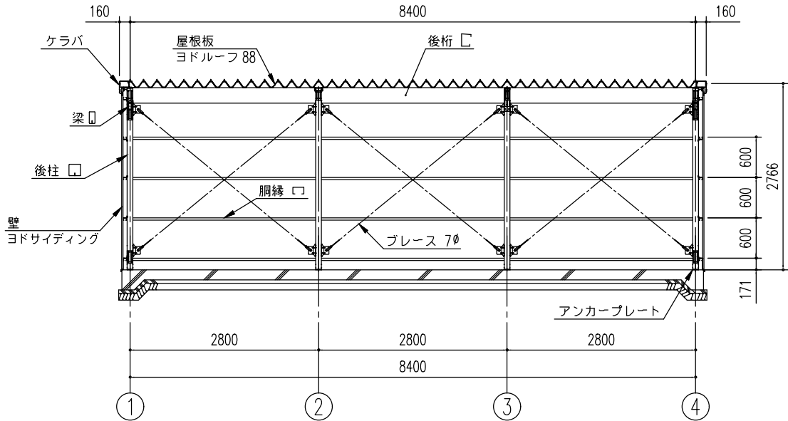
本体 正面断面図 (S= 1/80)
