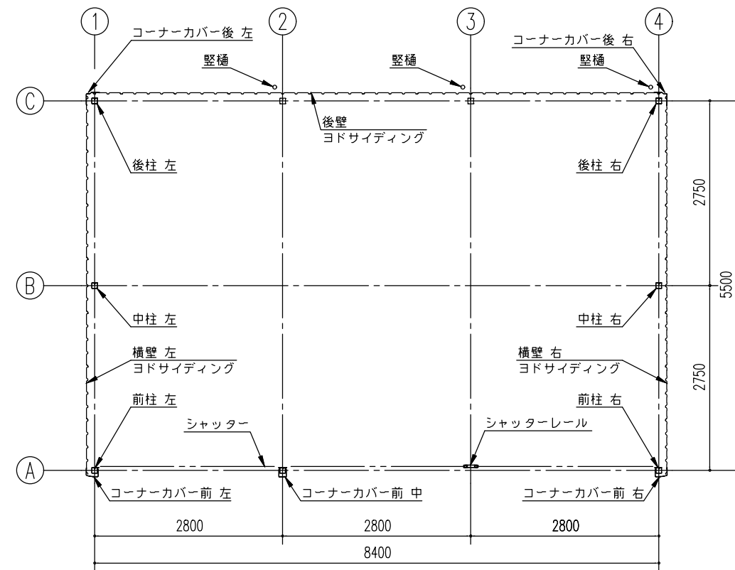
平面図 (S=1/80)
