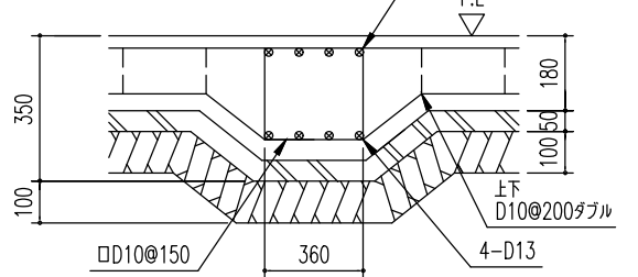
C ~ C' 断面
