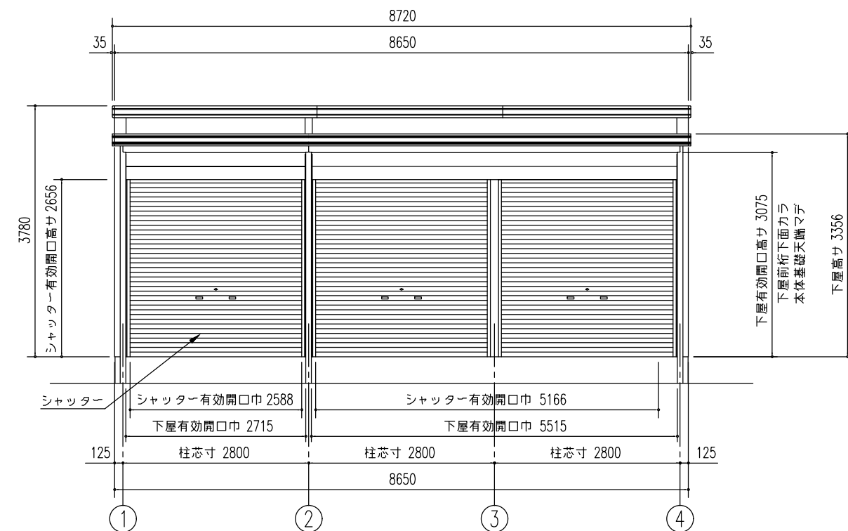
正面立面図(S=1/80)
