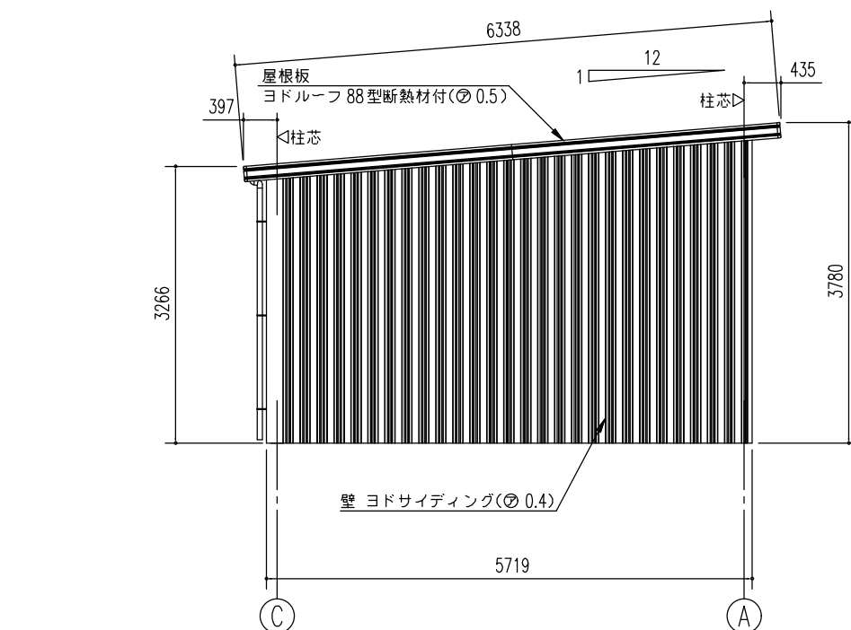
側面立面図 (S=1/80)
