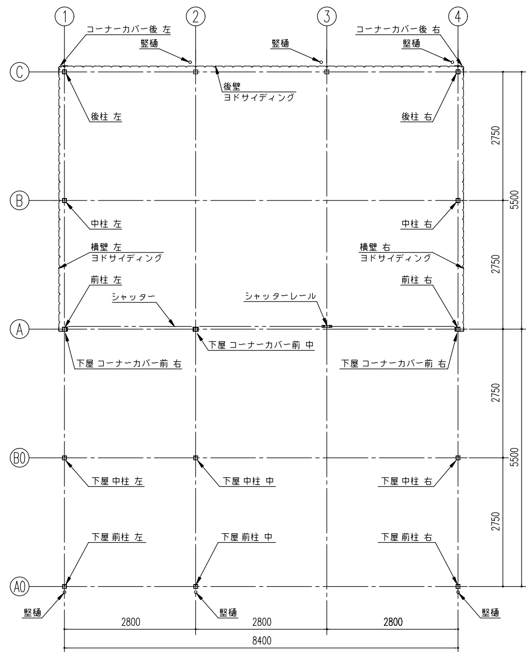
平面図 (S=1/80)
