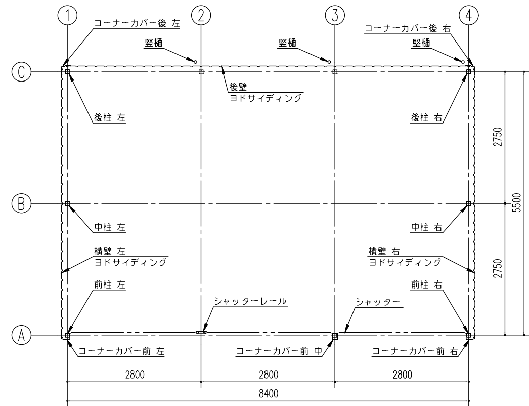
平面図 (S=1/80)
