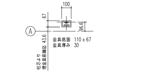
埋金具詳細図 ( S = 1/20)
