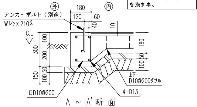
埋金具詳細図 ( S = 1/20)
