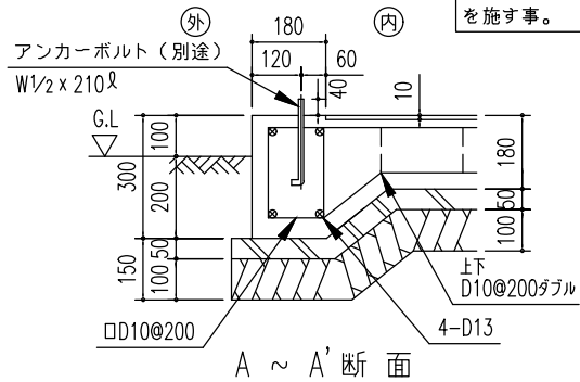
埋金具詳細図 ( S = 1/20)
