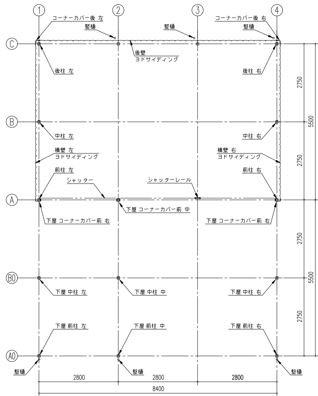
平 面 図 (S= 1/80)
