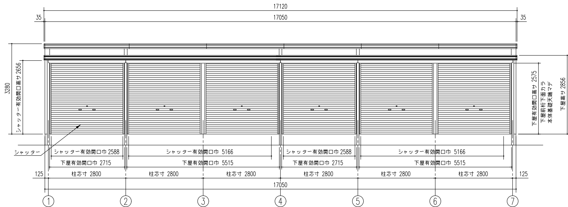
正面立面図(S= 1/80)
