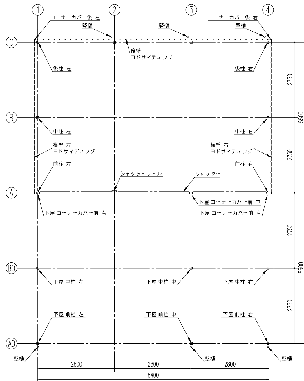
平面図 (S=1/80)
