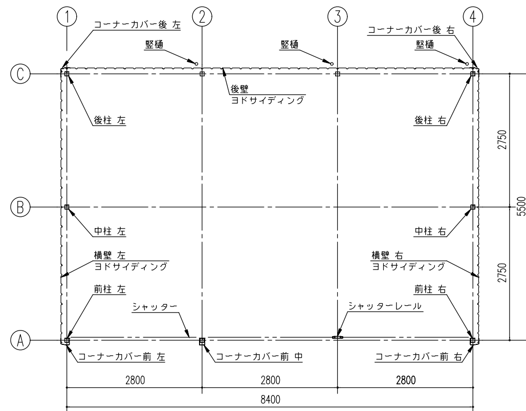
平面図 (S=1/80)
