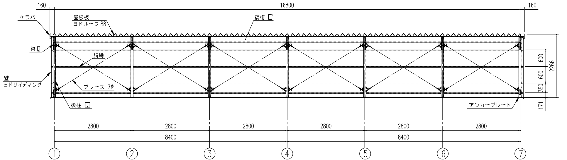
正面断面図 (S= 1/80)
