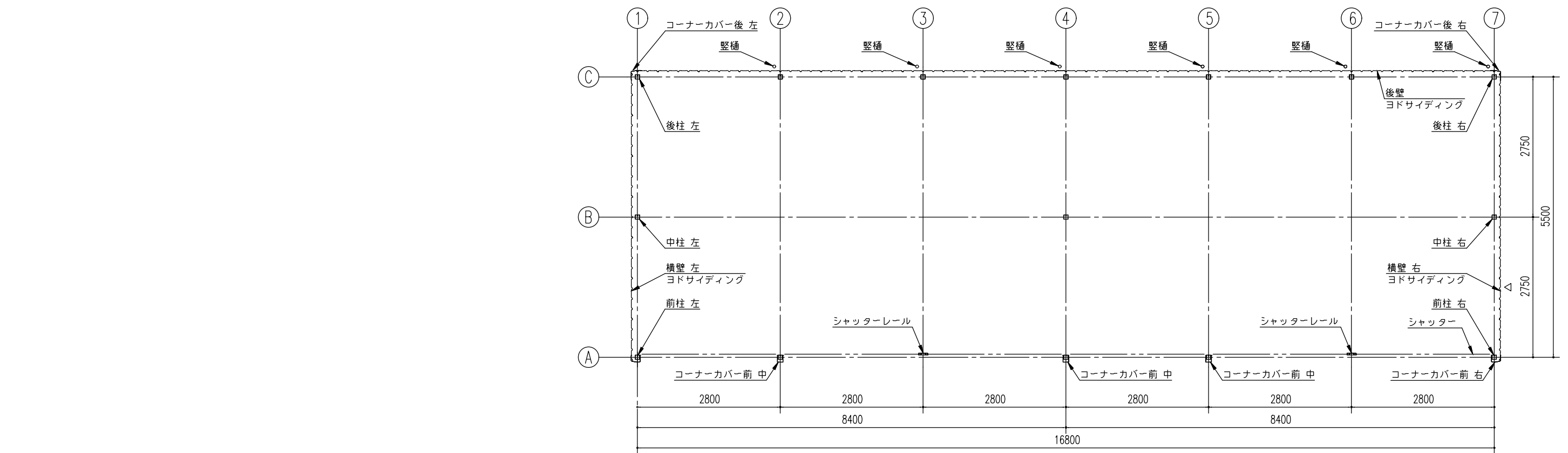
平面図 (S= 1/80)
