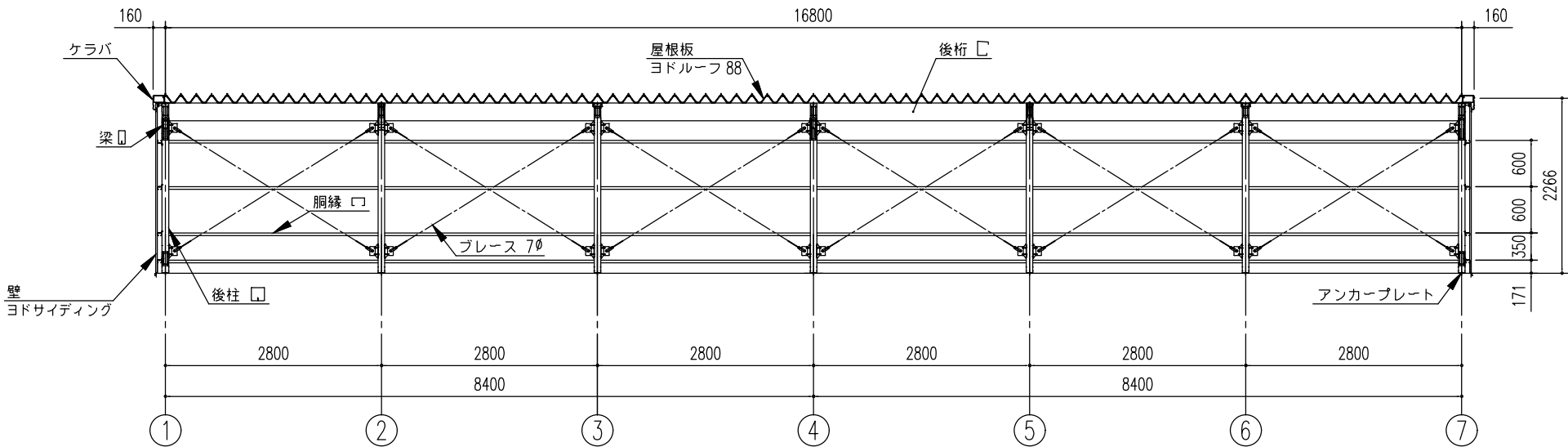
正面断面図 (S= 1/80)
