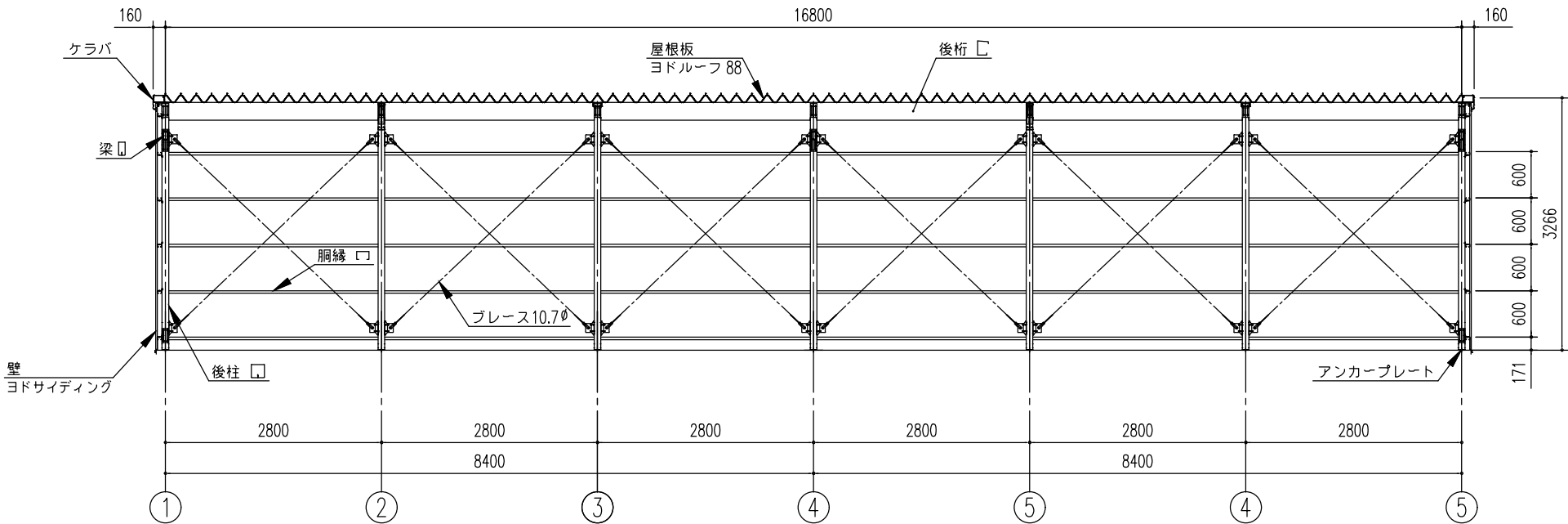
正面断面図 (S= 1/80)
