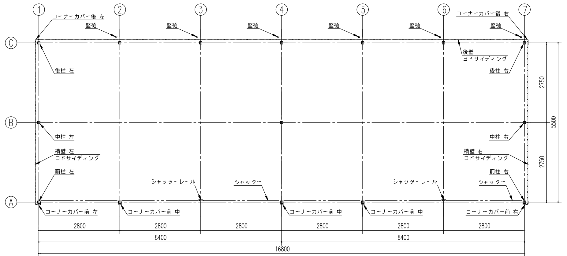
平面図 (S=1/80)
