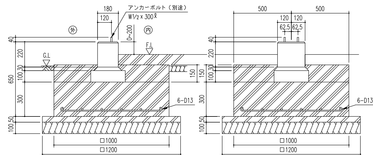
C ~ C' 断面
