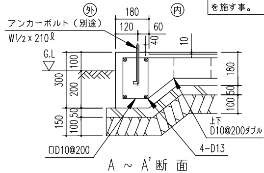
埋金具詳細図 (S= 1/20)
