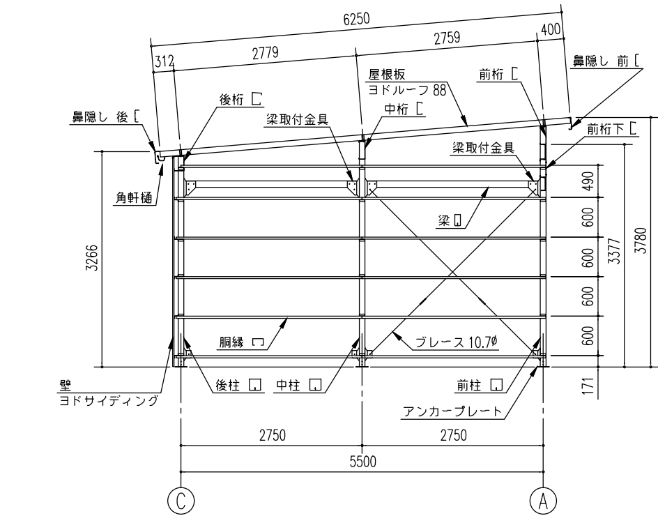
側面断面図 (S= 1/80)
