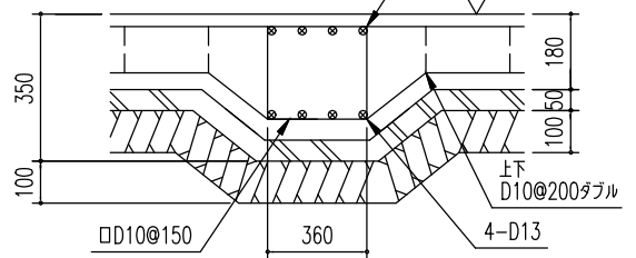
C ~ C'断面
