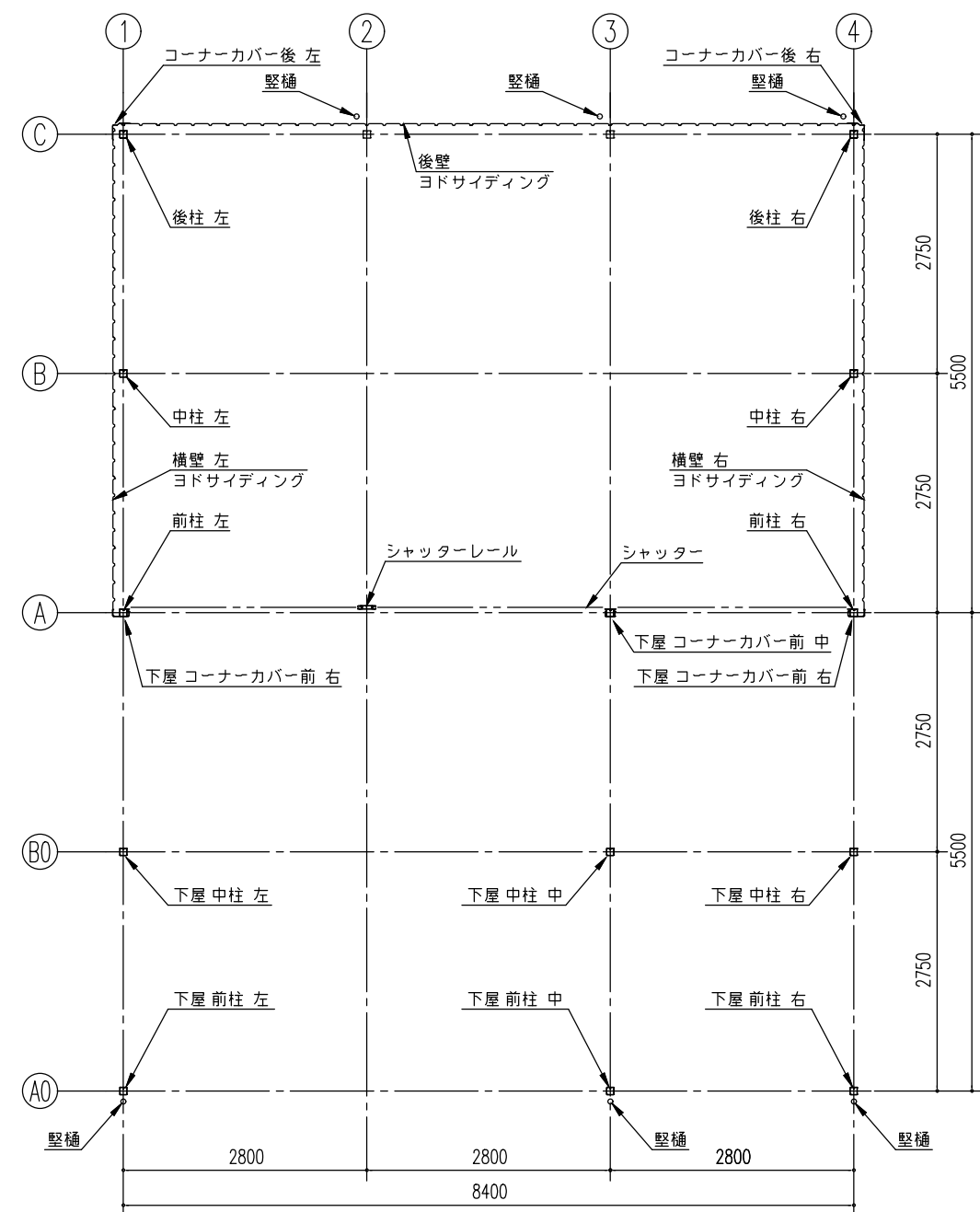
平面図 (S=1/80)
