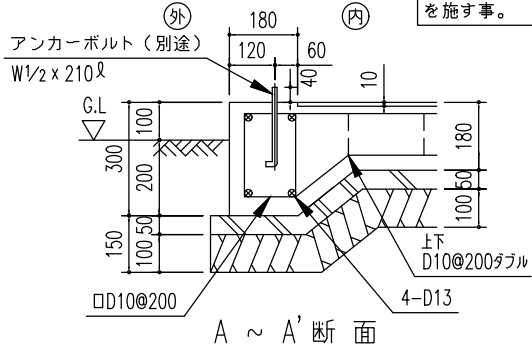
埋金具詳細図 ( S = 1/20)
