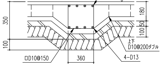
C ~ C' 断面
