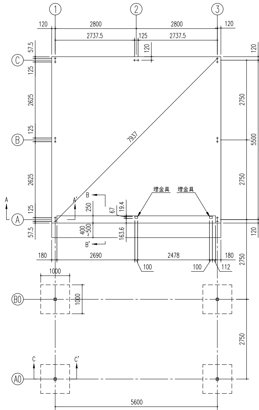
基礎伏図 (S=1/80)
