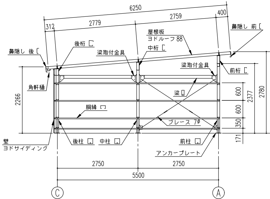
側面断面図 (S= 1/80) ※側面の出入口により、ブレースの配置が 変更となる場合があります。
