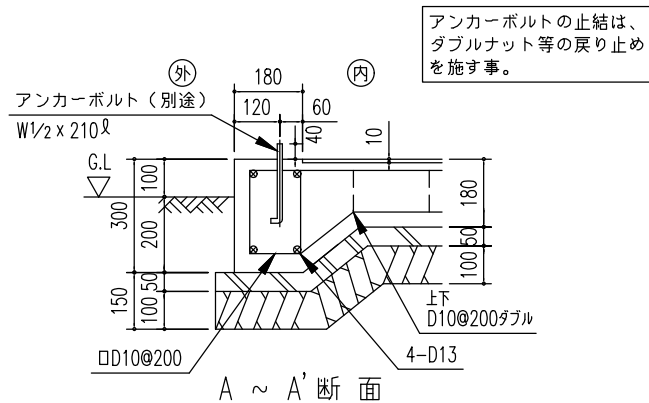
埋金具詳細図 (S = 1/20)
