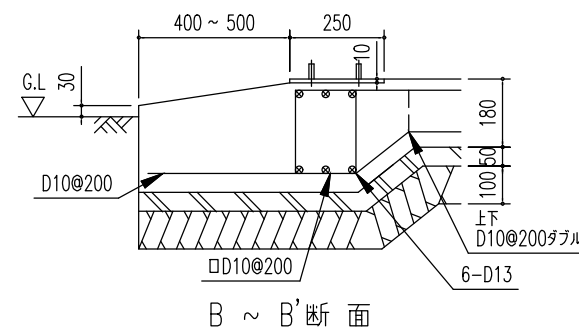
ベタ基礎断面図 (S=1/20)
