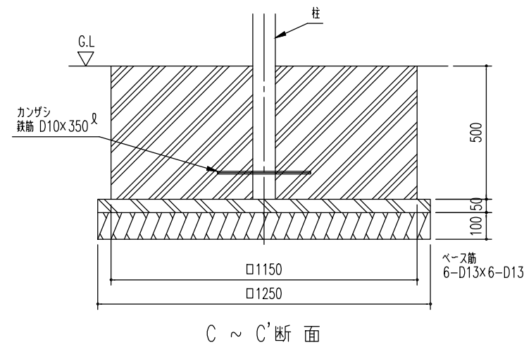
独立基礎断面図 (S=1/20)
