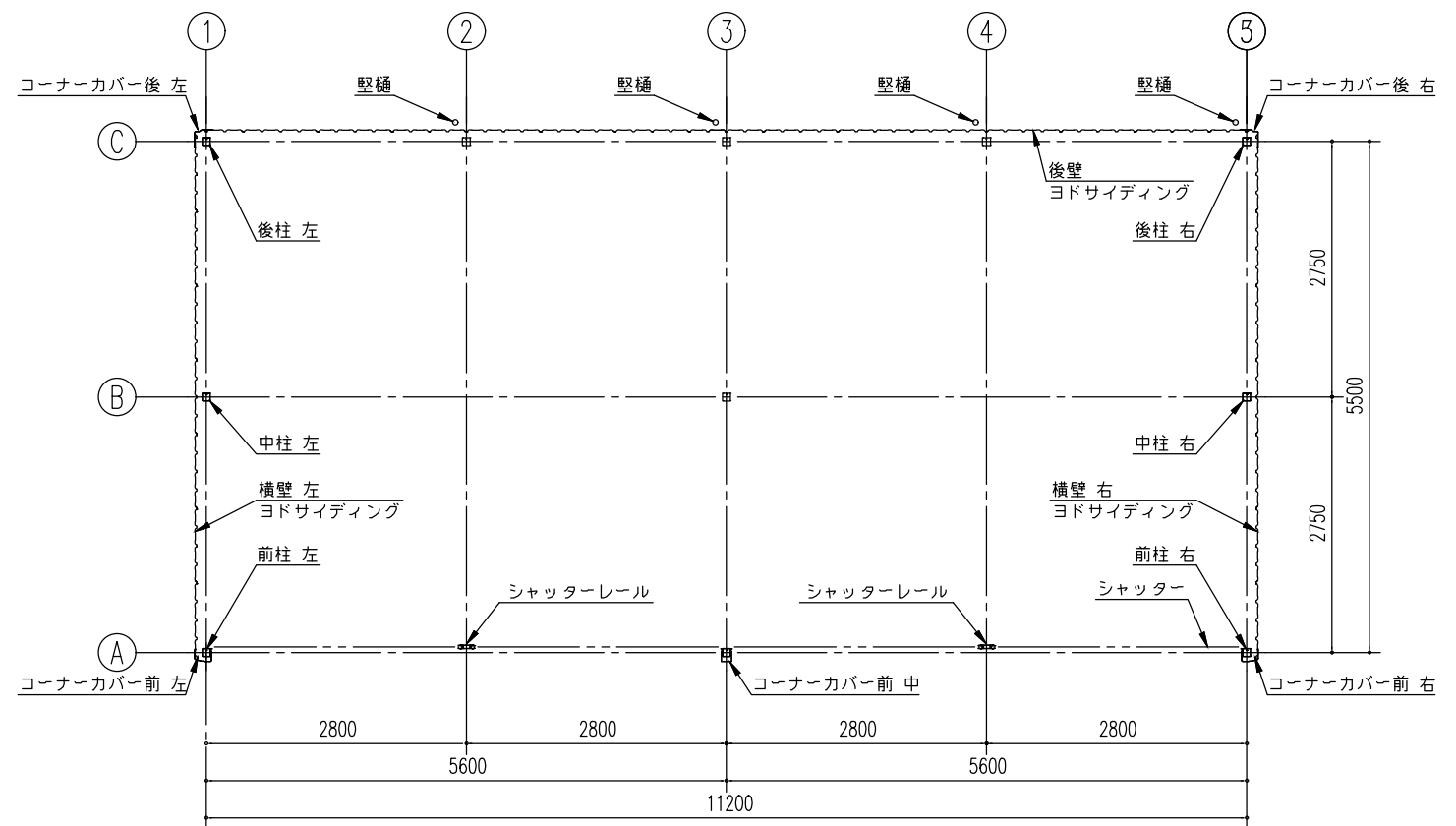
平面図 (S= 1/80)
