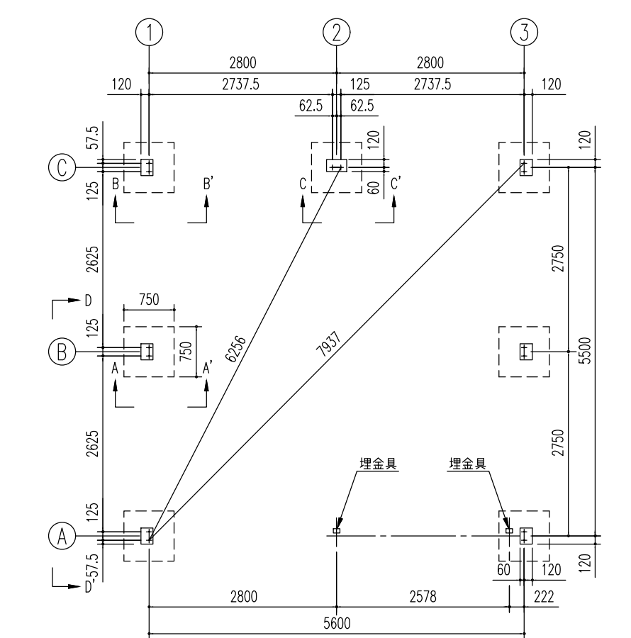
基礎伏図 (S=1/80)
