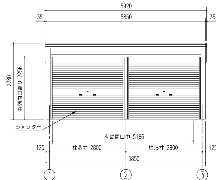
正面立面図 (S=1/80)
