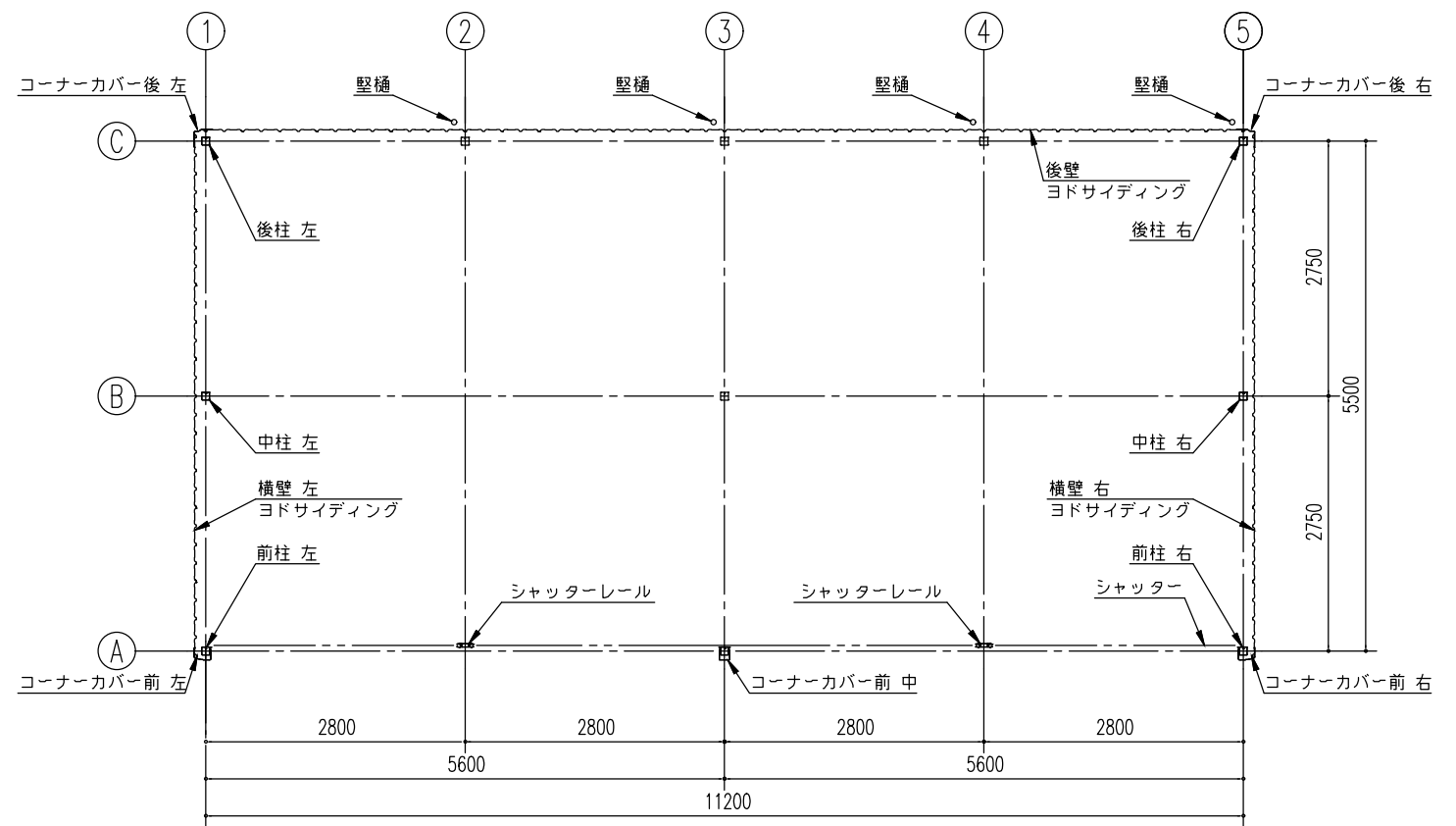
平面図 (S= 1/80)
