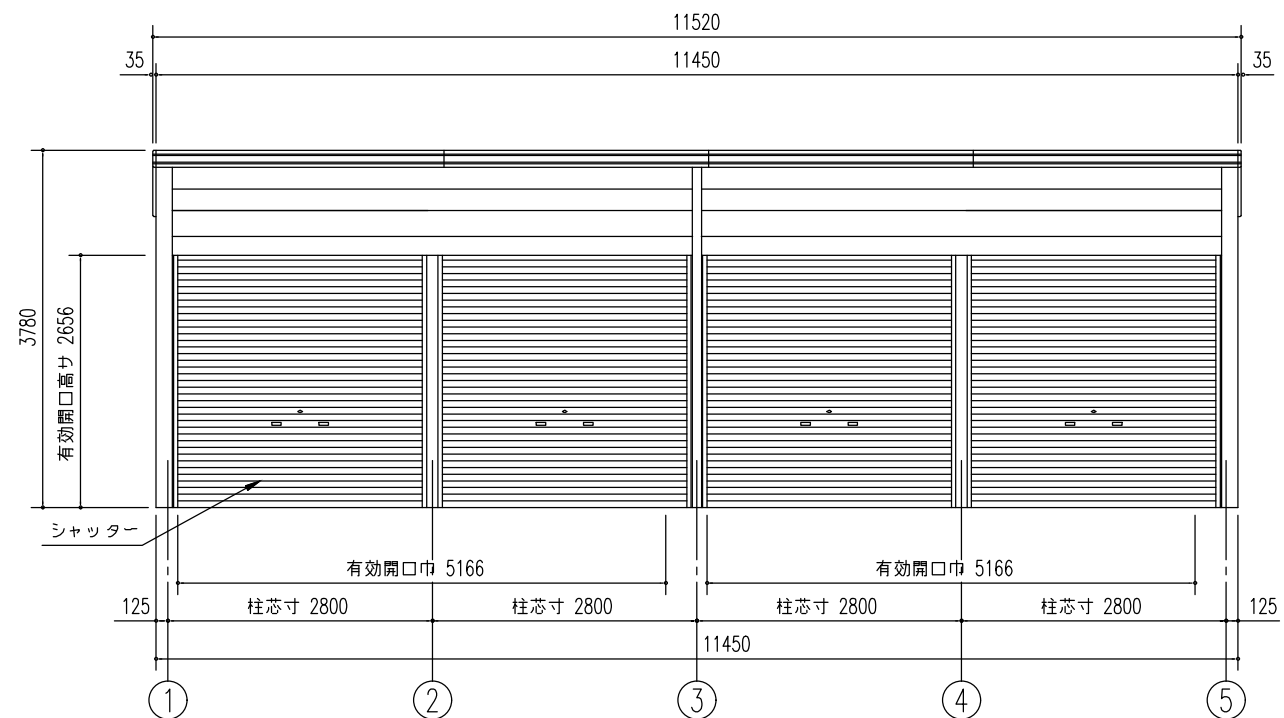
正面立面図(S= 1/80)
