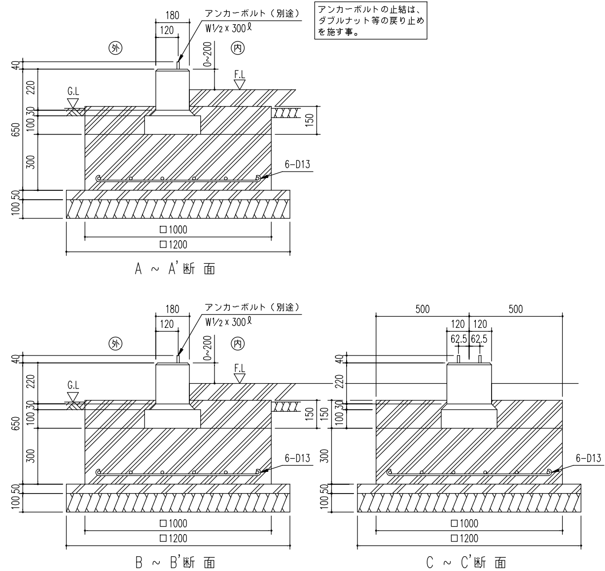
独立基礎断面図 (S=1/20) <下記条件での参考図> (地耐力 50 kN/m 2 以上, コンクリート設計基準強度 18 N/mm 2 以上) (基準風速 34 m/s, 地表面粗度区分 Ⅲ) 注1) 寒冷地の場合、凍結深度等を考慮し、実情にあわせて設計して下さい。 注2) 水切りを取り付けた際、光漏れの可能性がありますので基礎の立ち上がり部と天面部の角に面取りをしないでください。 注3) その他現地の実情にあわせて設計して下さい。
