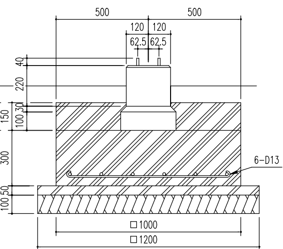
C ~ C' 断面
