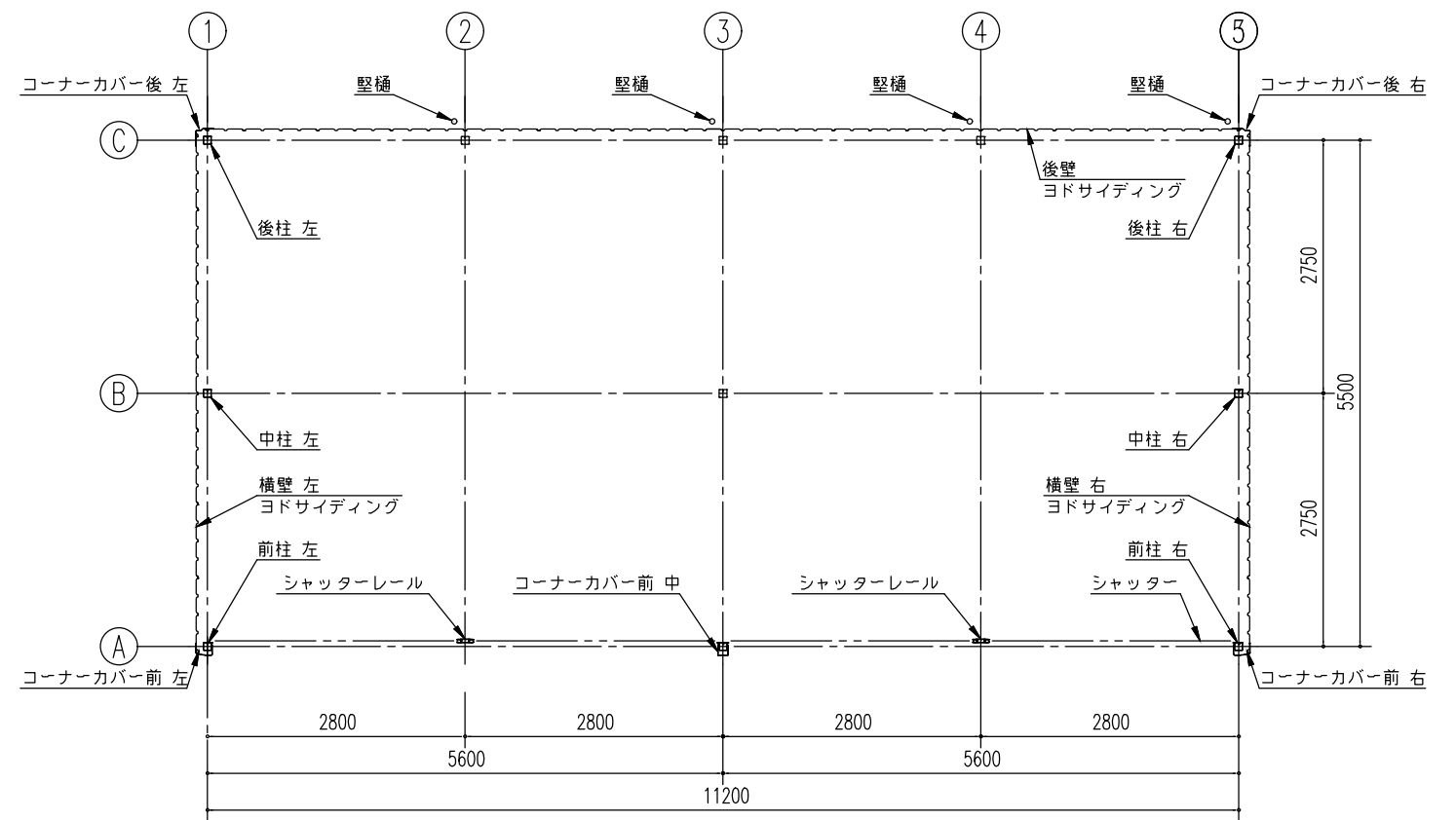
平面図 (S=1/80)
