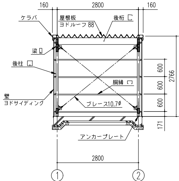
本体 正面断面図 (S= 1/80)
