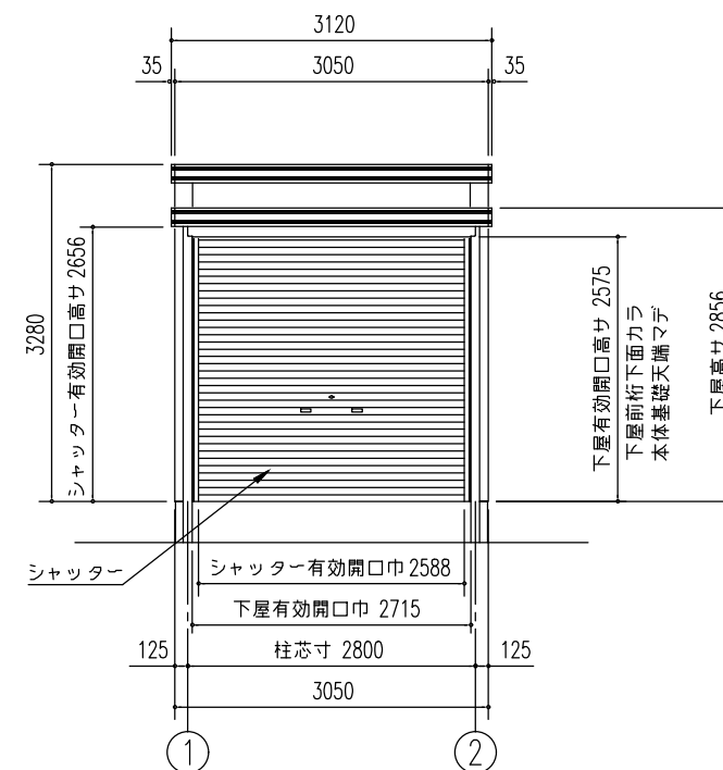
正面立面図 (S=1/80)
