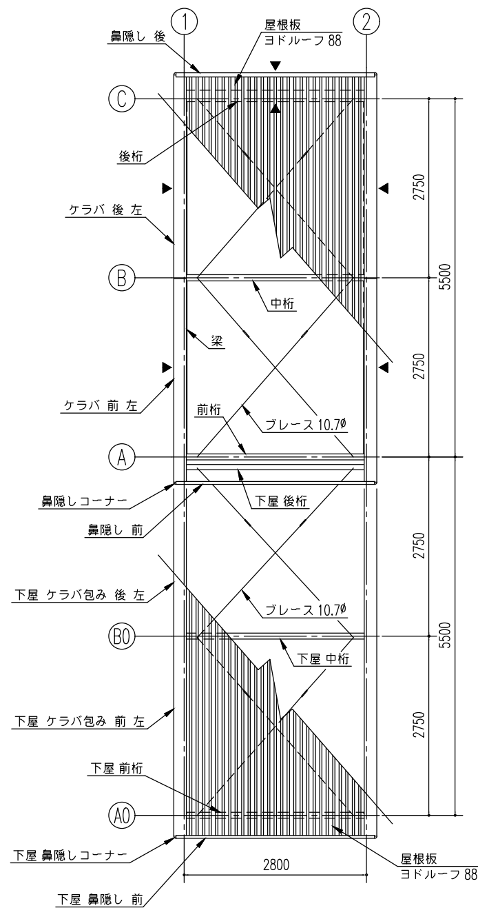
小屋伏図 (S=1/80) ▶は、ブレース 10.7φ とする。 ▶◀は、ダブルブレース 10.7φ とする。
