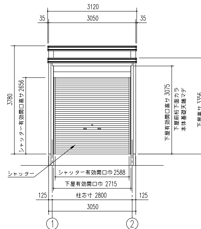
正面立面図 (S=1/80)
