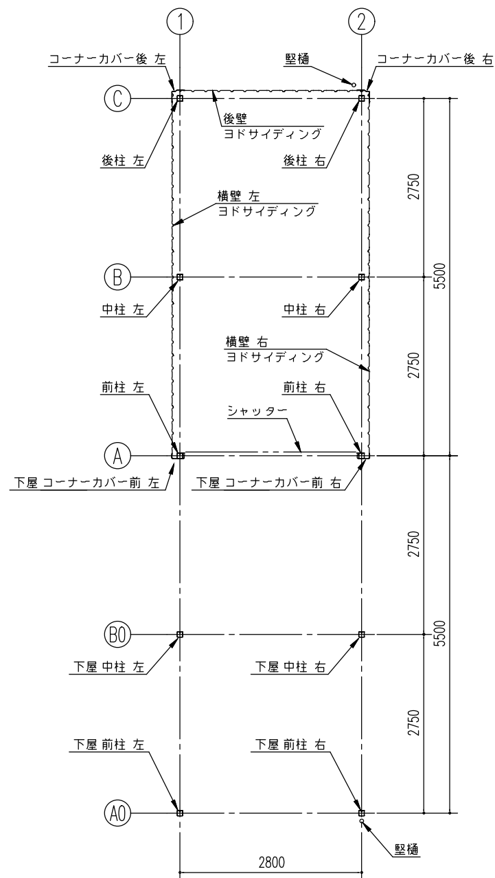
平面図 (S=1/80)
