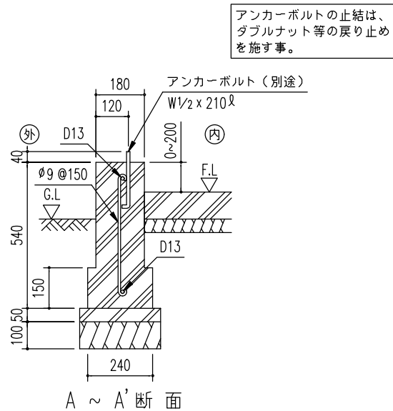
布基礎断面図 (S = 1/20)
