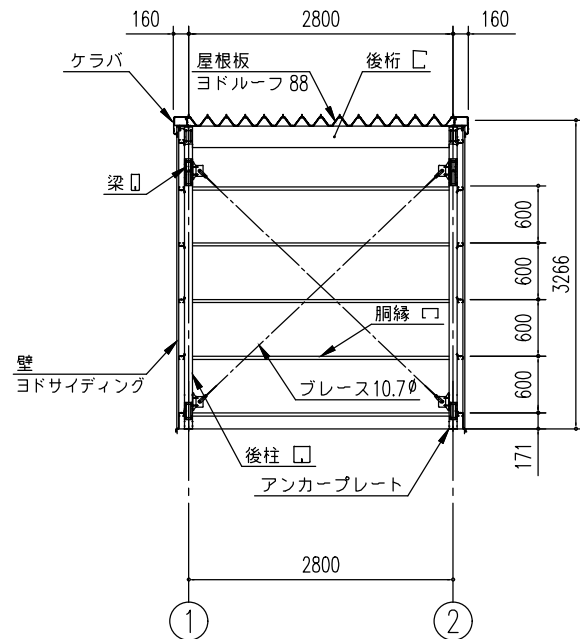
正面断面図 (S= 1/80)
