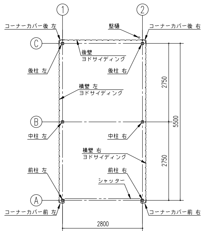
平面図 (S=1/80)
