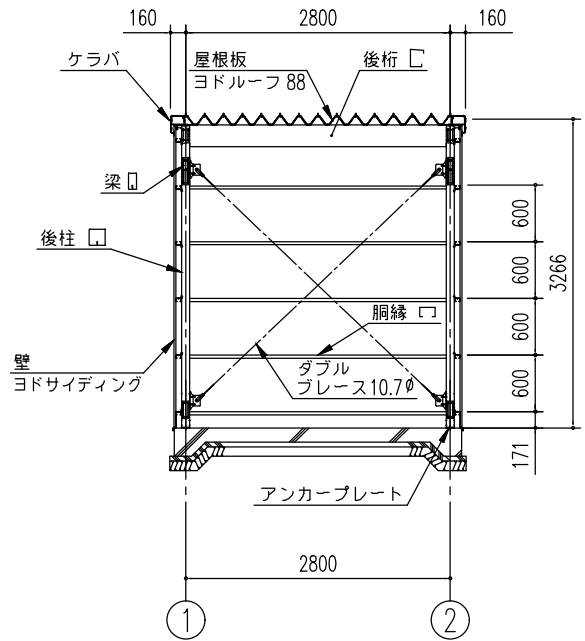
本体 正面断面図 (S= 1/80)
