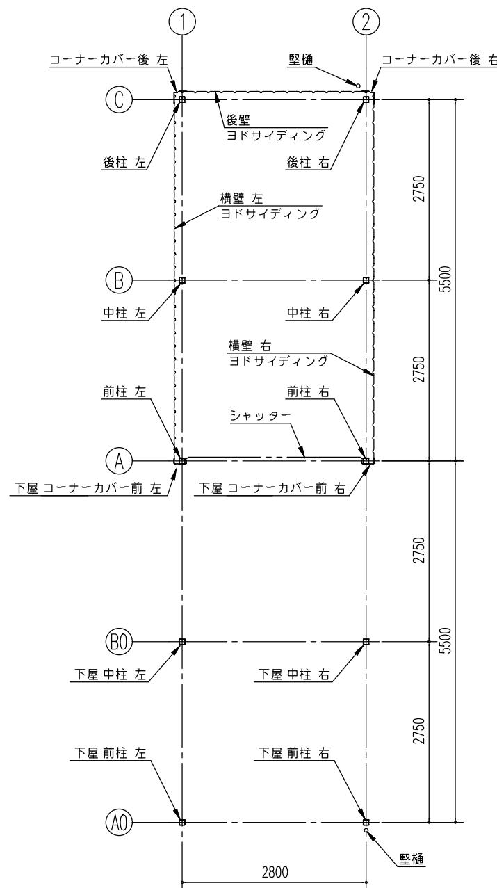
平面図 (S=1/80)
