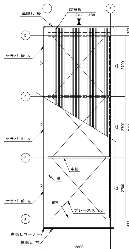
小屋伏図 S=1/80
