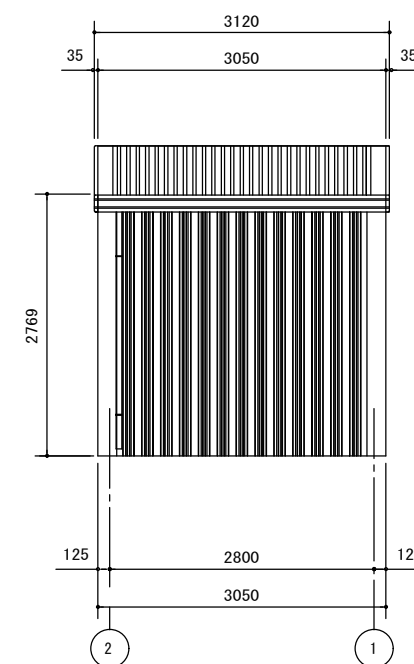
後面立面図 S=1/80
