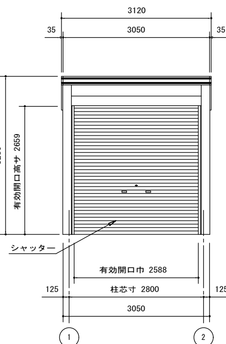
正面立面図 S=1/80
