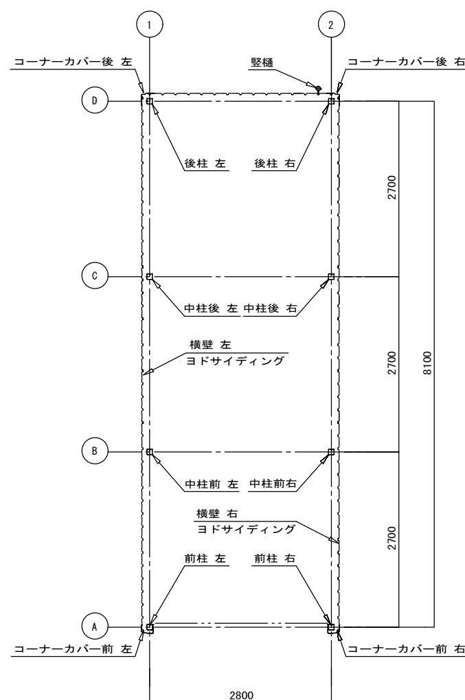
平面図 S=1/80
