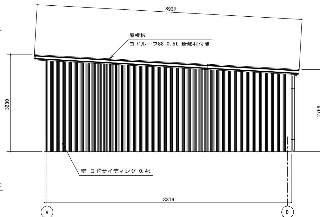
側面立面図 S=1/80
