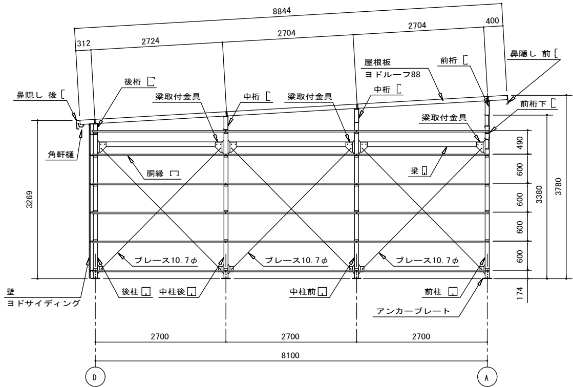
側面断面図 S=1/80
