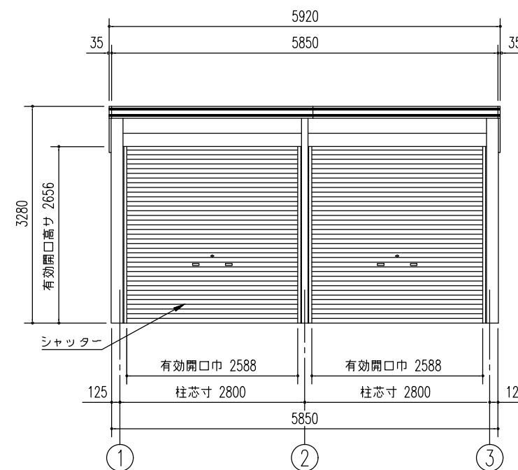
正面立面図 (S=1/80)
