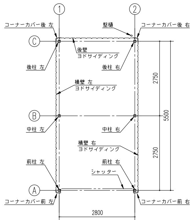
平面図 (S=1/80)
