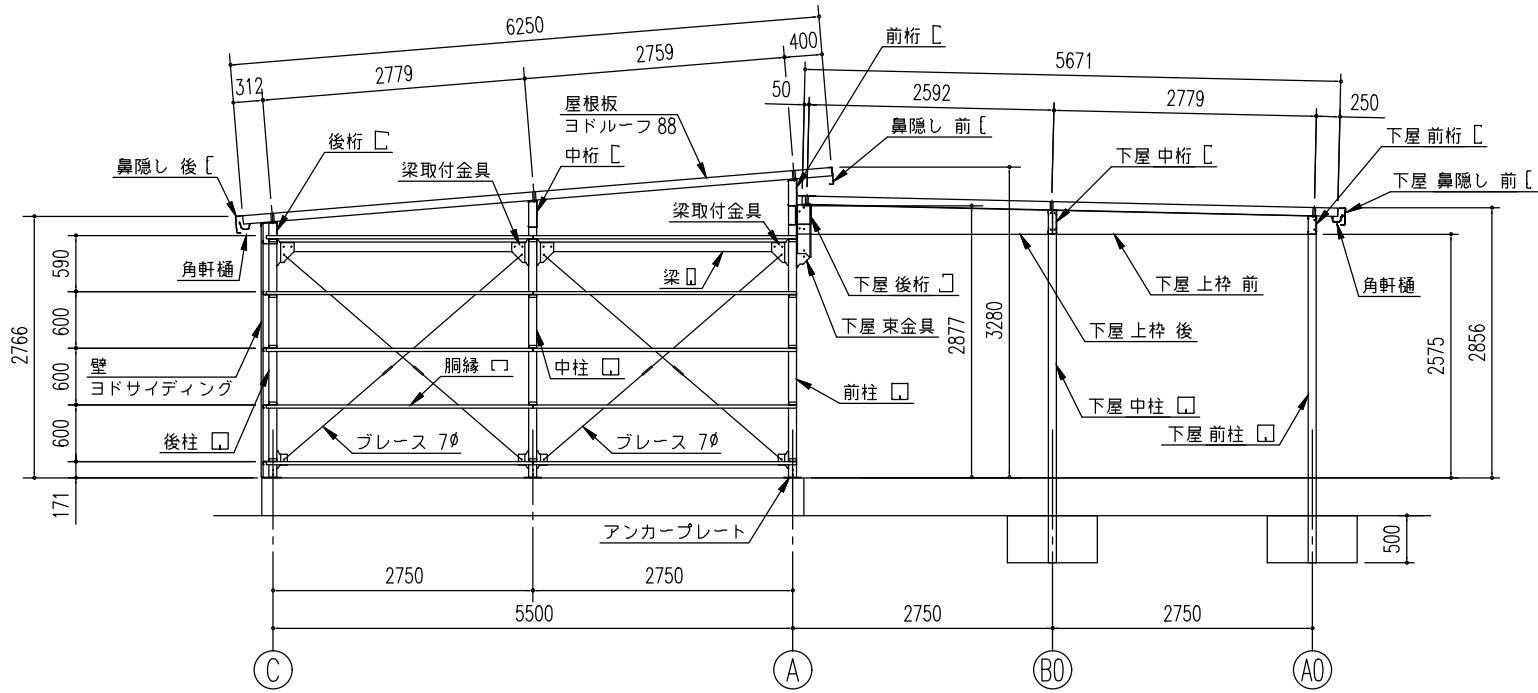
側面断面図 (S= 1/80) ※側面の出入口により、ブレースの配置が 変更となる場合があります。
