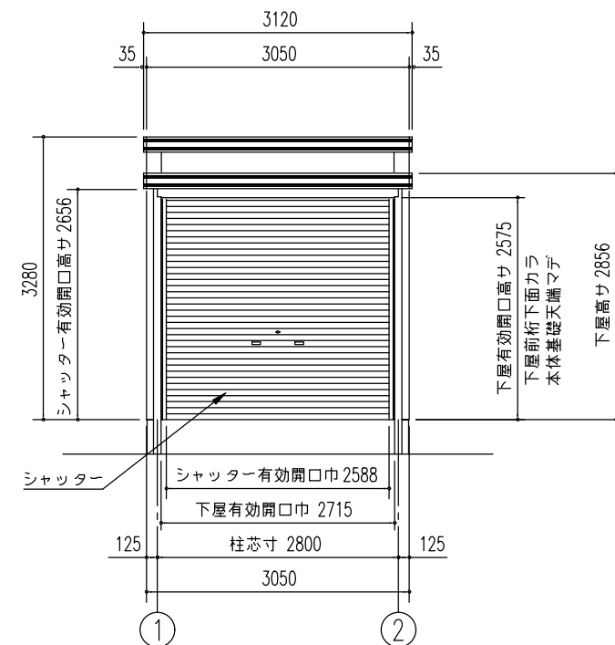
正面立面図 (S=1/80)
